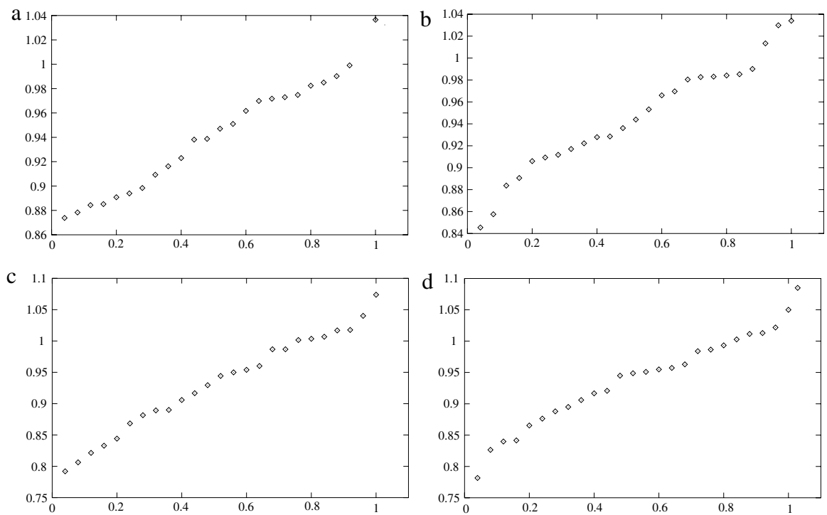
Fig. 2. The marginal scaled TTT transform of (a) T_1^{-1} , (b) T_2^{-1} , (c) T_3^{-1} , and (d) T_4^{-1} .
