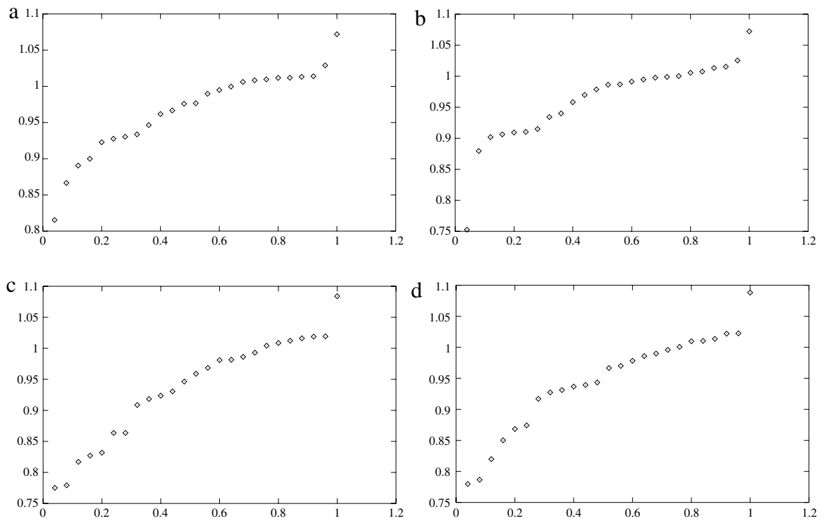
Fig. 1. The marginal scaled TTT transform of (a) T_1 , (b) T_2 , (c) T_3 , and (d) T_4 .
