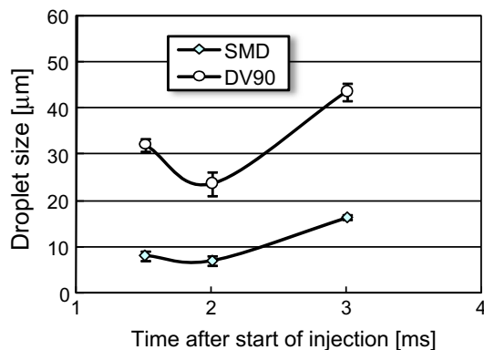
(b) P_a = 0.4 MPa
