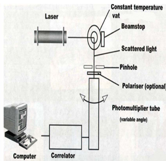
(d) Photon Correlation Spectroscopy
