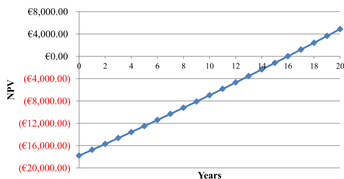
Fig. 14. NPV with ELF 1 kW.
